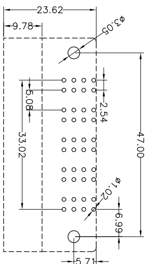
P.C.B Layout
